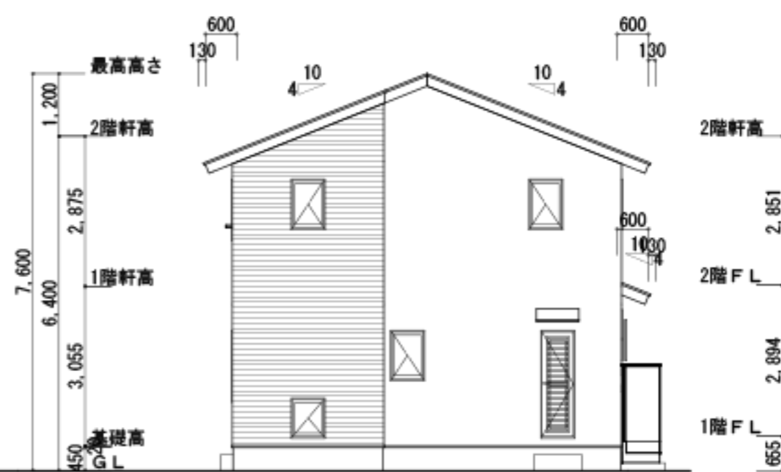
東側立面図
