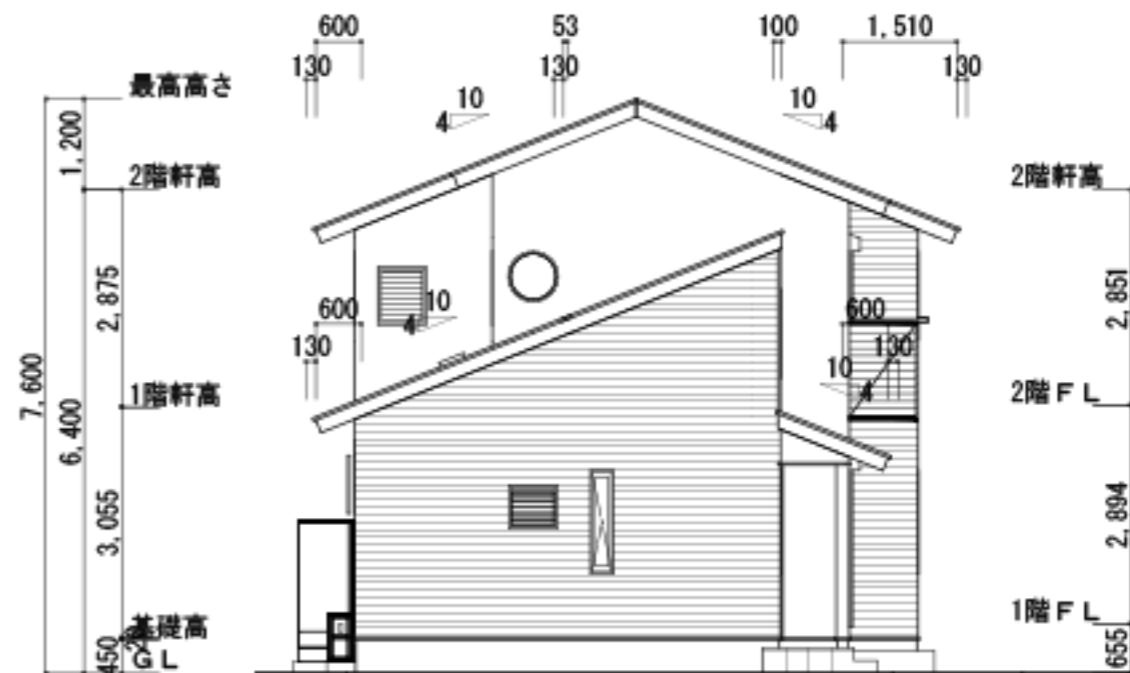
西側立面図
