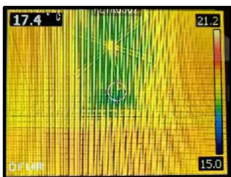
小屋裏からエアコンの冷気が落ちている様子 38坪の住宅を市販のエアコン1台のみで 住宅全体を冷やしている
