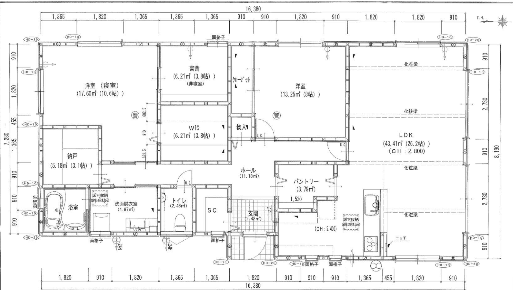
平面詳細図 S:1/50
